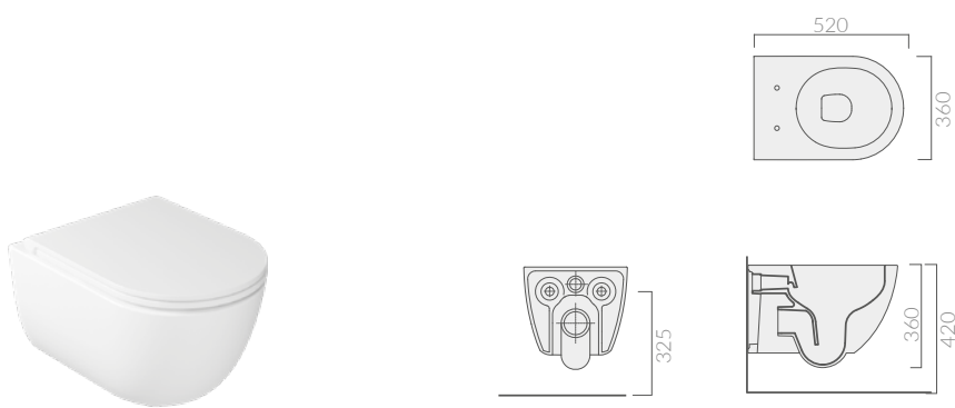
Wc sospeso SENZA BRIDA 52x36 cm.
