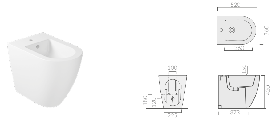
Bidet monoforo 52x36 cm, fissaggio a scomparsa incluso.
