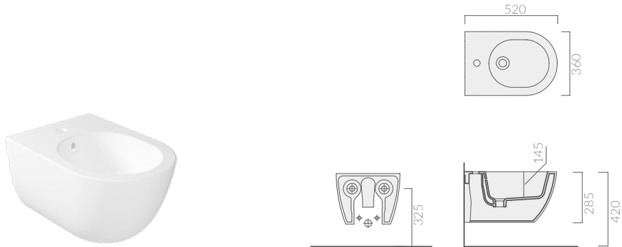
Bidet sospeso monoforo 52x36 cm.
