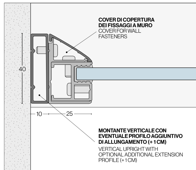
SEZIONE PROFILO A MURO DALL'ALTO WALL PROFILE SECTION FROM ABOVE
